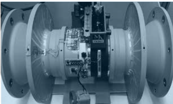
Arbre de transmission
